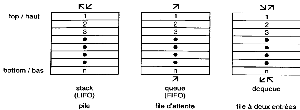
Figure 1 – Stack, queue, and dequeue Figure 1 – Pile, file d'attente et file à deux entrées
